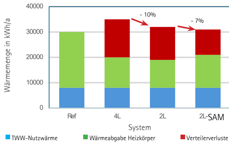
Energiebedarf Gesamtgebäude
